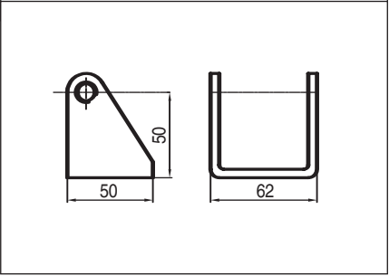
Окраинная скоба алюминиевая (прилагается бесплатно)
