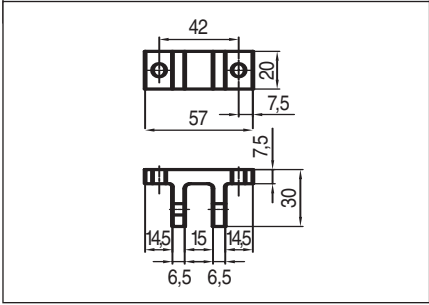
Крепеж стержневой для подвижной створки (прилагается бесплатно)
