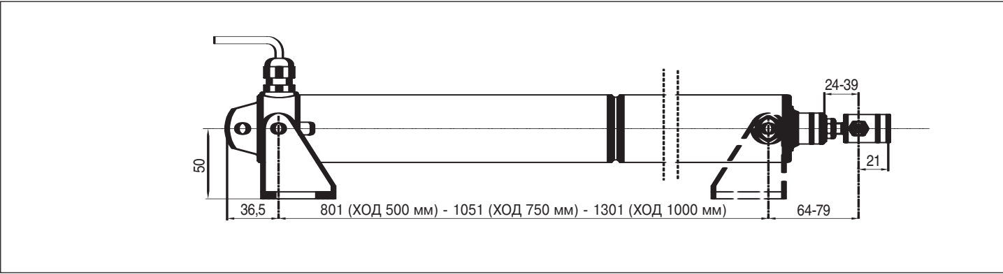
Размеры движка
