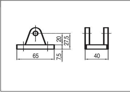
Крепежная алюминиевая скоба для заднего крепления код 80382I
